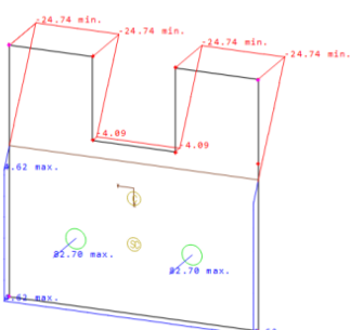
Contraintes à l'ELU
