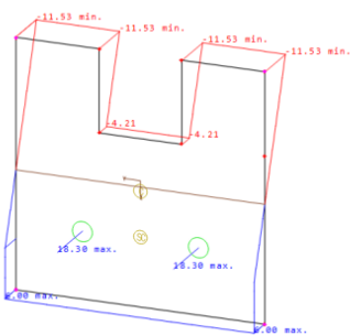
Contraintes à l'ELS
